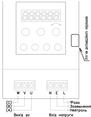
Мал. 1. Схема електричних з'єднань.
