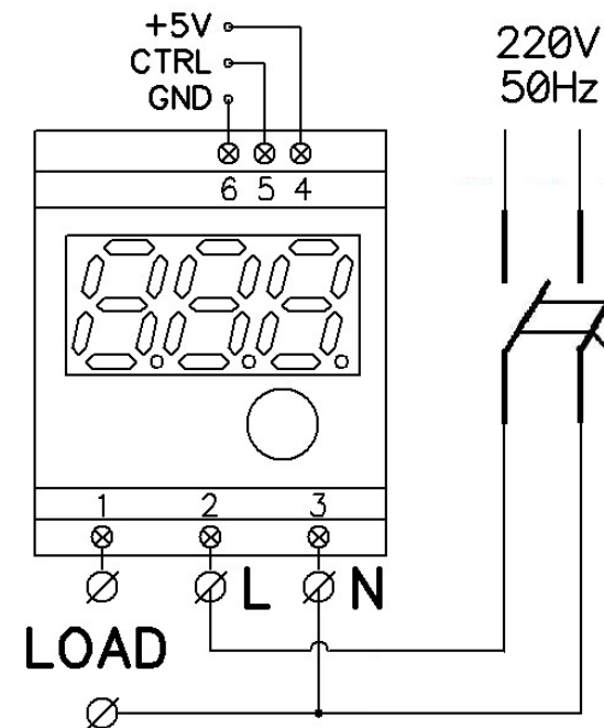
Мал. 1. Схема електричних з'єднань.
